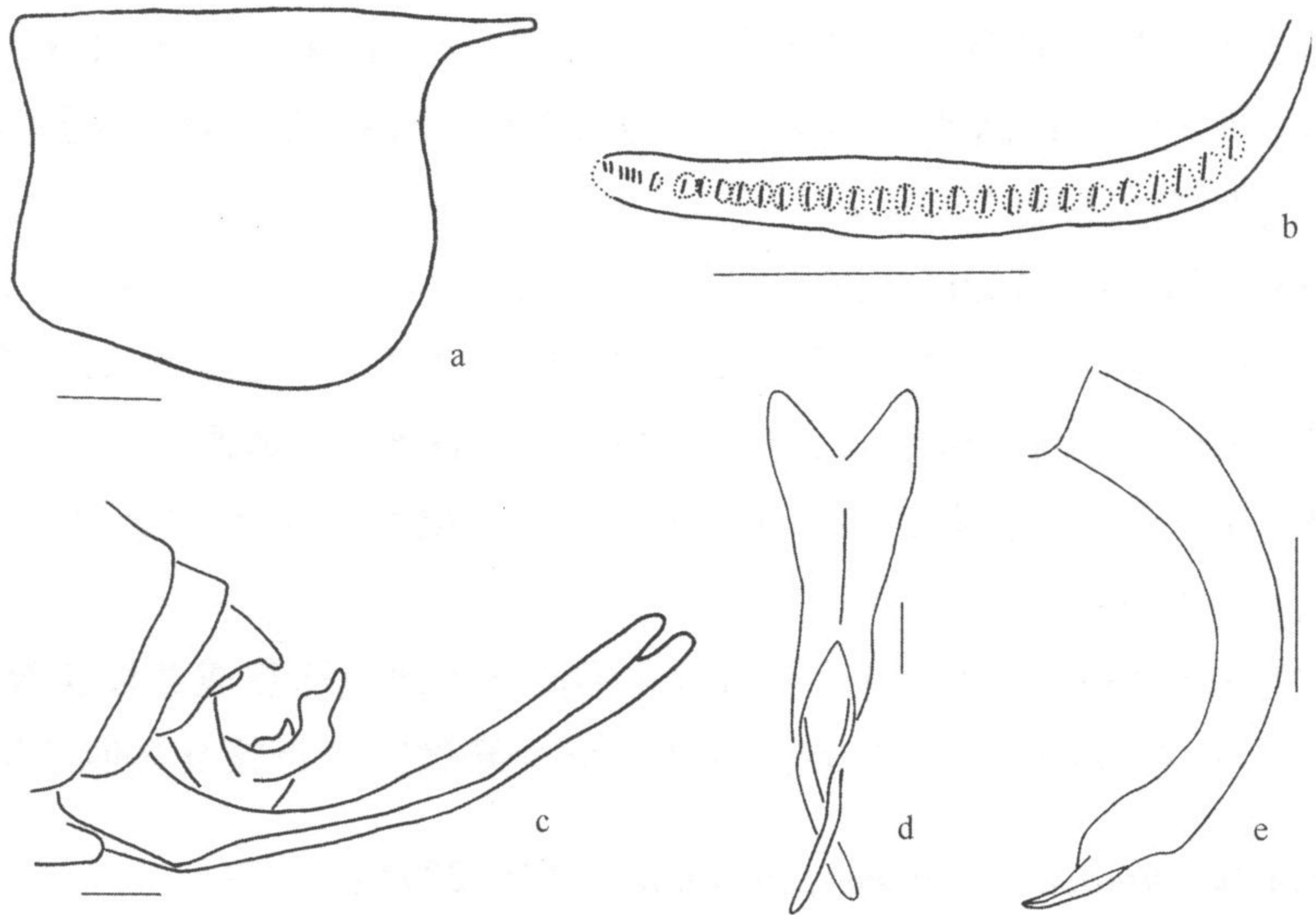
图 224 异舰掩耳螽 Elimaea (Elimaea) paranautica Liu
